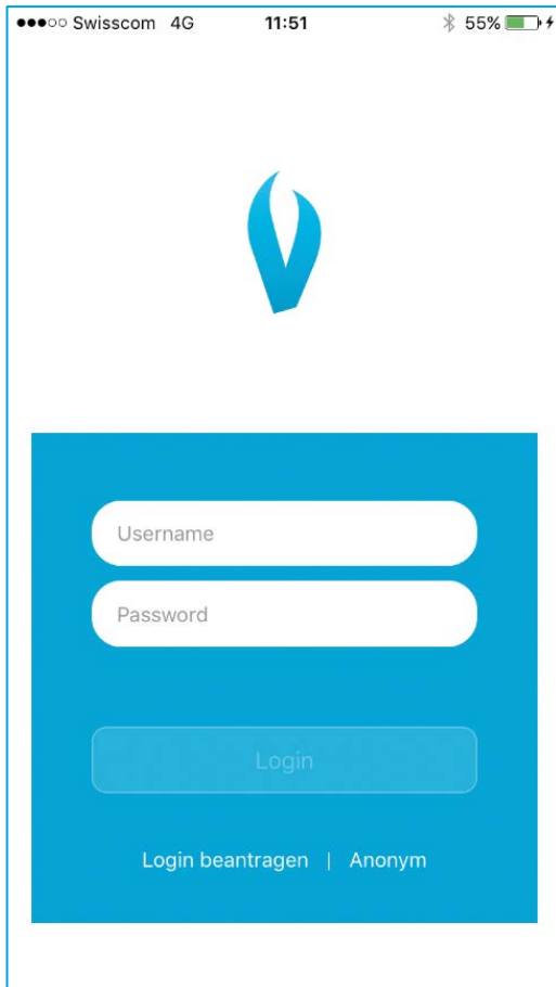
Abbildung 1 Login
